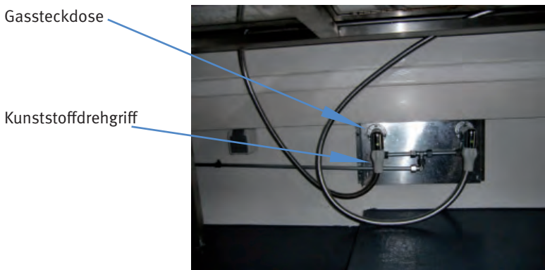
Abb. 20: Beispielhafte Edelstahl-Geflecht-Schlauchleitung mit Kunststoffdrehgriff und Gassteckdose
