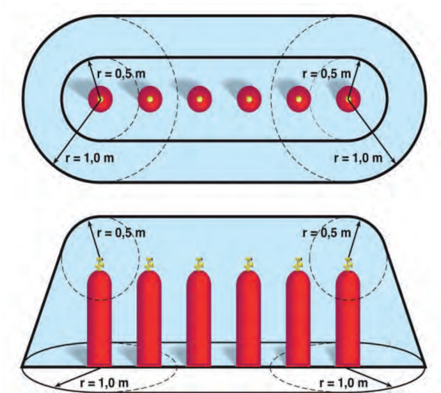
Abb. 8: Schutzbereiche für Mehrflaschenanlagen mit 2 bis 6 Flaschen im Freien: 0,5 m um jede Anschluss- stelle und kegelförmig bis zum Boden, am Boden r = 1\text{ m}
